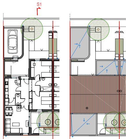
HABITATGE TIPUS-1 PLANTA.
