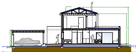
SECCIÓ-2
