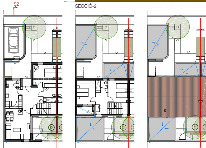
HABITATGE TIPUS-2 PLANTES
