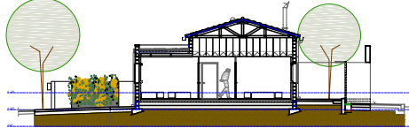
SECCIÓ-1
