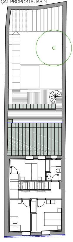
PLANTA SEGONA PROPOSTA
