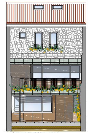
ALÇAT PROPOSTA JARDÍ
