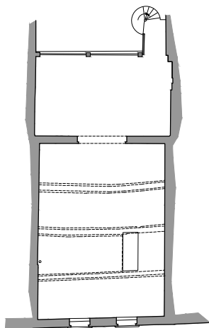
PLANTA PRIMERA ACTUAL
