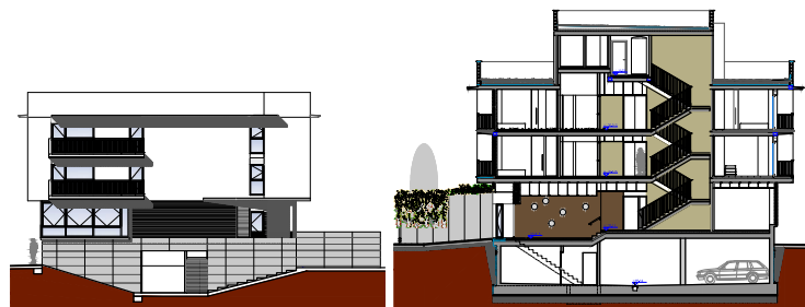
ALÇAT SUD
