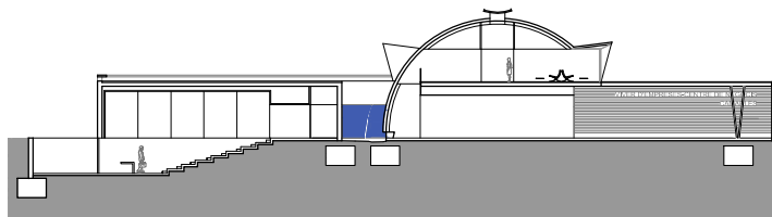
SECCIÓ 1-1'
